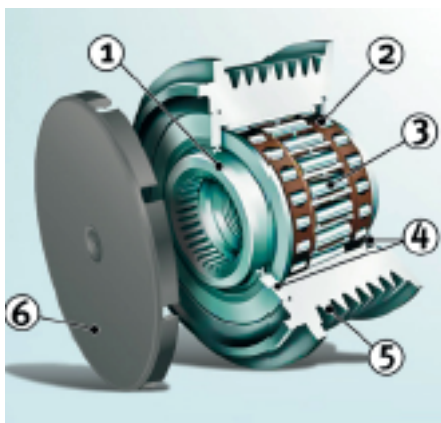
Foto 4: Sprzęgiełko alternatora
